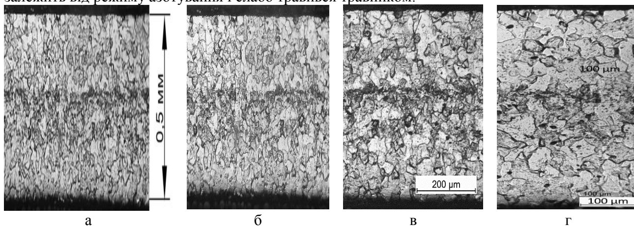
Рисунок 2 – Макроструктура зразка №1 із титатного сплаву ВТ1-0 в поздовжньому перетині по товщині листа
