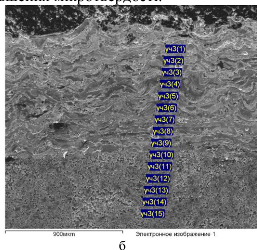
Рисунок 1 – Результати кількісного стереологічного аналізу пористості (а) та структура (б) поверхні з напиленим покриттям після електроконтактної обробки
