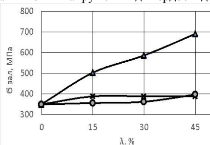
Рисунок 3 – Залежність залишкових напружень від ступеня деформації сталі 40ХНМА:
